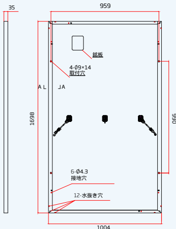
背面図
